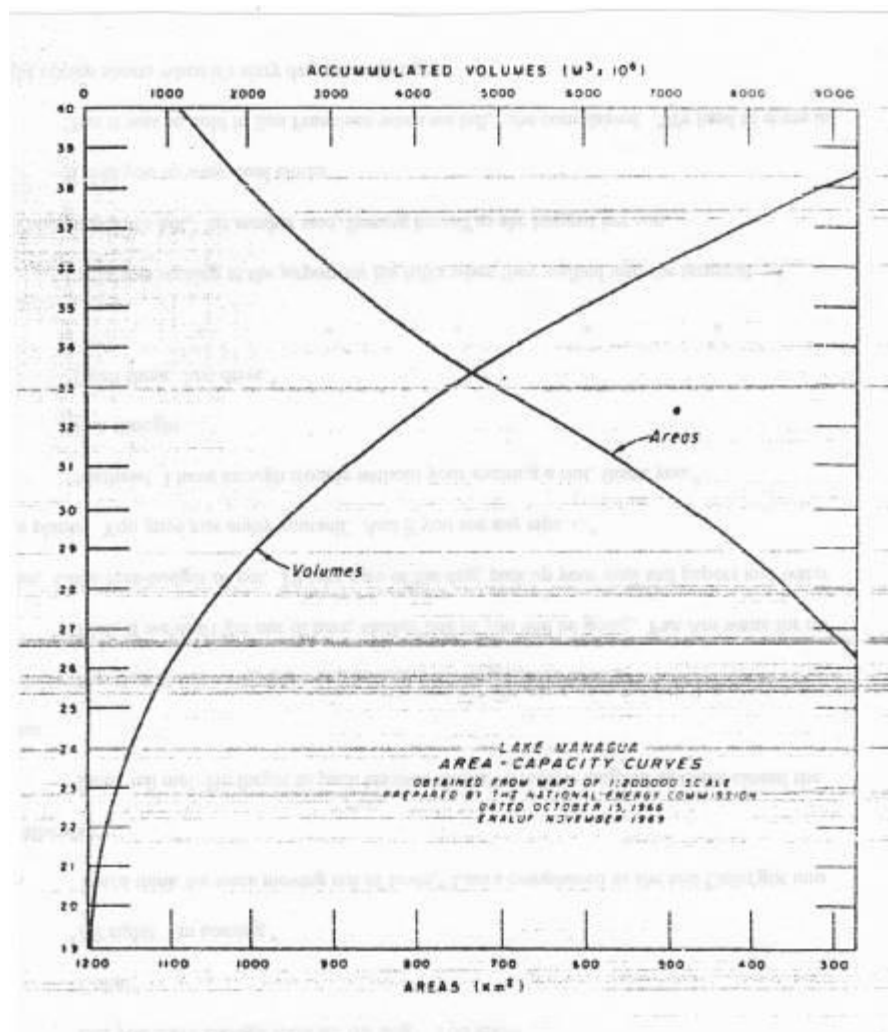
Area y Capacidad vs nivel del lago Xolotlán
