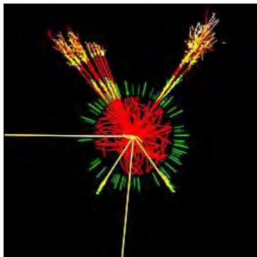
Producción simulada por ATLAS de un evento de Higgs en el Large Hadron Collider en CERN. El evento se produce cuando dos protones chocan y se producen cuatro muones cuyas trayectorias se muestran en amarillo.
