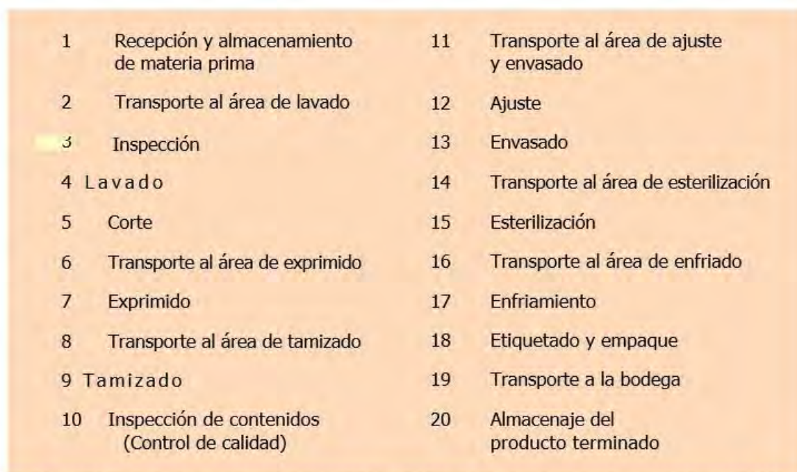
Figura 18. Flujo de proceso para industria de jugo de naranja en una mediana empresa. Fuente: (41)
