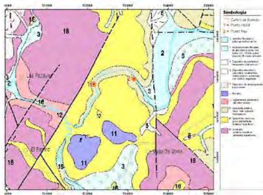
Mapa geológico del Cañón de Somoto. (Fuente: CzechAid/2004)
