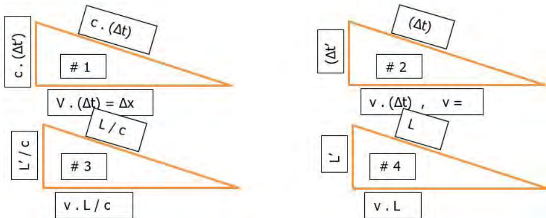
Figura 7. Las 4 versiones del mismo triángulo se obtienen al multiplicar las dimensiones por el mismo factor de proporcionalidad ( 1/c ). También en triángulos "3" y "4" " \Delta x " ha sido substituida por " L ". Aplicando el Teorema de
