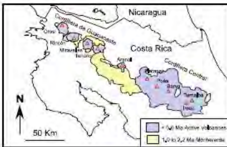
Figura 5. Mapa del frente volcánico activo y el frente volcánico de Monteverde en Costa Rica.
