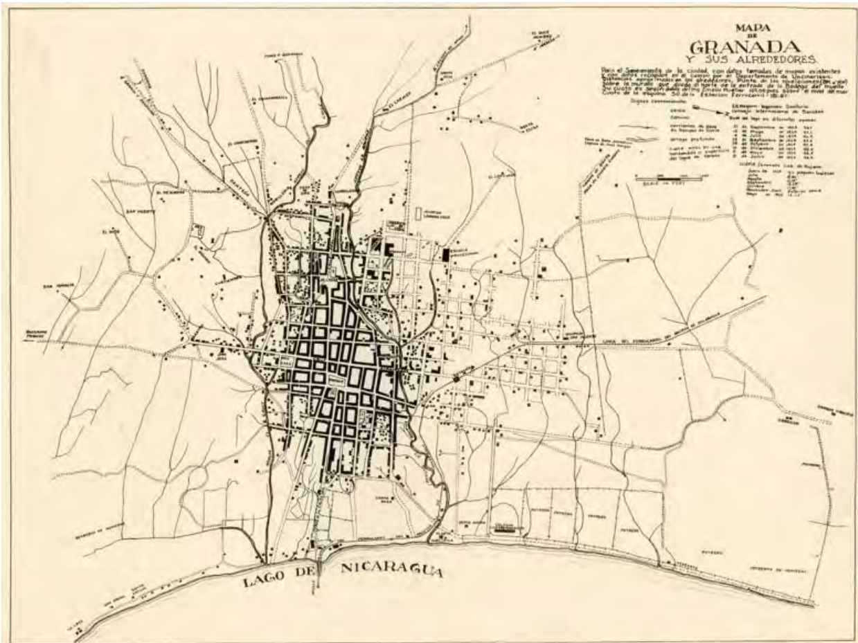
Mapa levantado por las autoridades sanitarias (uncinariasis), basado en mapas existentes, circa 1926. Reproducimos la leyenda para beneficio del lector.
