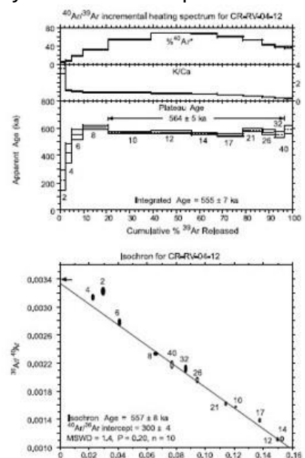
Figura 3. Espectros de calentamiento escalonado para la muestra CR-RV-04-12 del volcán Rincón de la Vieja. Los pasos de calentamiento, en vatios, están escritos debajo de los pasos de liberación de Ar en el diagrama de meseta y junto a las elipses de error en el diagrama de isócrona inversa. Pasos 2 y 4 vatios no incluidos en isócrona.
